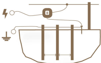
Obrázek č. 10: Přepětové ochranné zařízení s bleskojistkou
